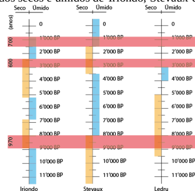
Figura 05: Gráfico analítico referente as descrições de períodos secos e úmidos de Iriondo, Stevaux e Ledru
